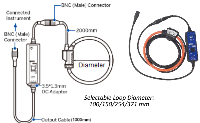
PMSC-SCCP-5kA-500mV
