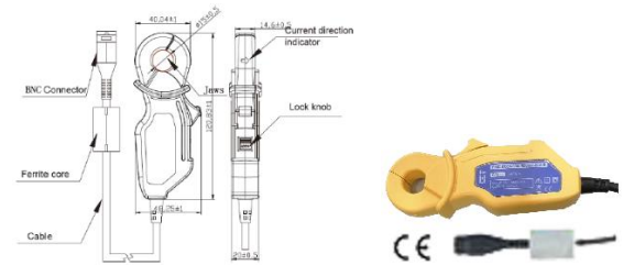
PMSC-SCCP-50A-500mV
