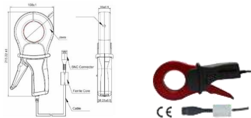
PMSC-SCCP-500A-500mV
